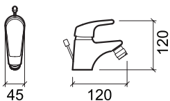
5360400 misturadora de bidé c/ VDA bidet mixer w/ pop up waste mitigeur de bidet a/ vidage
