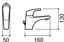
5364300 misturadora de lavatório sénior c/ VDA senior basin mixer w/ pop up waste mitigeur de lavabo senior a/ vidage
