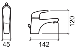
5360300 misturadora de lavatório c/ VDA basin mixer w/ pop up waste mitigeur de lavabo a/ vidage
