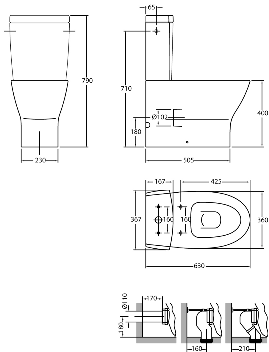
Inodoro BTW tanque bajo de alimentacion lateral
