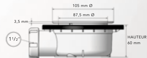
BONDE SIPHOÏDE receveur de douche
