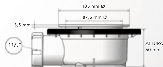
VÁLVULA SIFÓNICA
