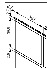
Detalle decorado Fresh de 120 cm
