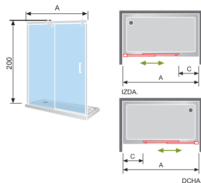
Ref. LM102 + LATERAL FIJO LM103
