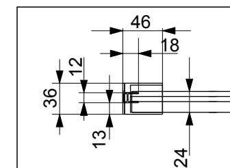
GS100 Lado fijo
