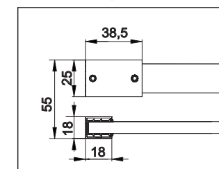
Lado fijo LM100 Frente de ducha
