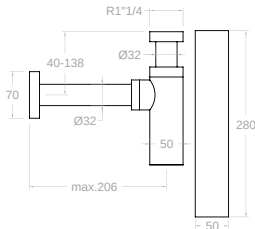
4790 212118 Sifón latón Brass siphon
