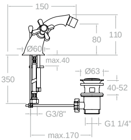
3103CVA1167 261830 Bimando para lavabo, con válvula automática. Ref. 1167 latón Twin handle bidet tap with pop up waste. Ref. 1167 brass
