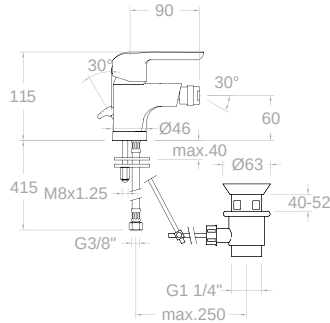
6603VA9065 240729 Monomando para bidé con válvula automática 1 1/4 ". Ref. 9065 ABS Bidet mixer with pop-up waste 1 1/4 ". Ref. 9065 ABS
