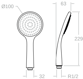
3521NL 241377 Ducha de mano con 1 función 1 function handshower
