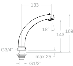
74302S 74Z301676 Cuerpo giratorio para caño fundido 743012 Moving head without spout for 743012
