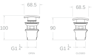
4719L 213477 Valvula de latón para desagüe sistema Quick Clac Quick Clac waste brass
