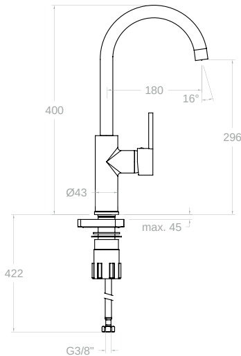
330602 33E301596 Monomando para fregadero con caño giratorio Wash basin mixer with swivel spout
