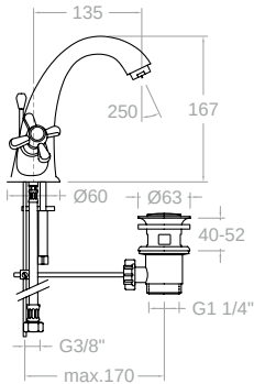
3101CVA1167 261828 Bimando para lavabo, con válvula automática 1 1/4" Ref. 1167 latón Twin handle wash basin tap with automatic valve Ref. 1167 brass
