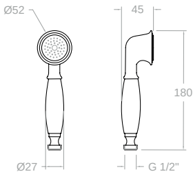
1224 179232 Ducha de mano de laton con 1 función 1 function handshower brass
