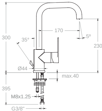
360302VA9065 36B303690 Monomando lavabo (S) con válvula automática 1 1/4\"/>
