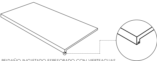
PELDAÑO INGLETADO ESPESORADO CON VIERTEAGUAS
