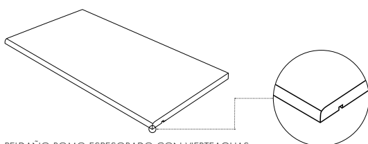
PELDAÑO ROMO ESPESORADO CON VIERTEAGUAS
