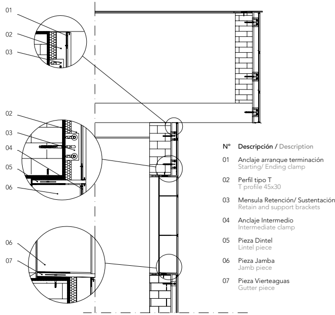
Componentes del sistema y soluciones técnicas System components and technical solution
