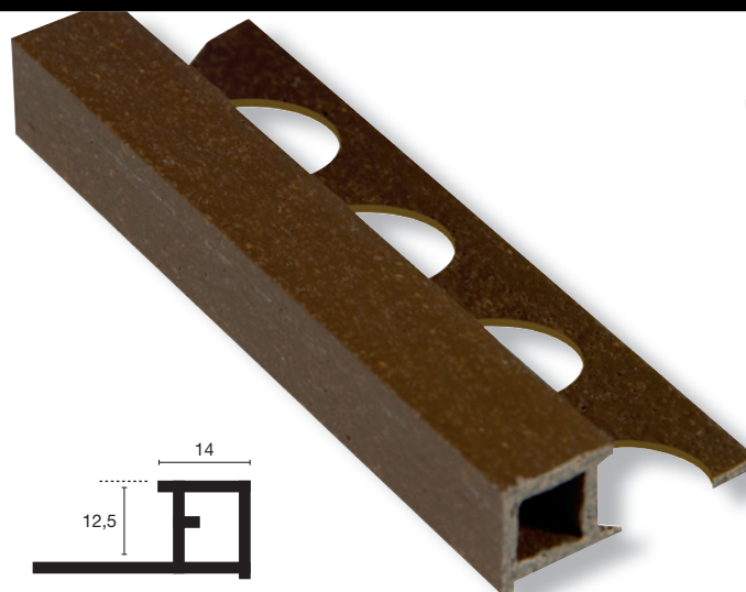
LISTELO RÚSTICO 12,5x14 MM. RUSTIC LISTELO 12,5x14 MM.
