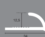
perfil rústico rustic profile
