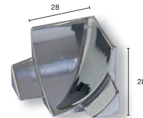
Conector Ref. 1 • 2 conexiones
