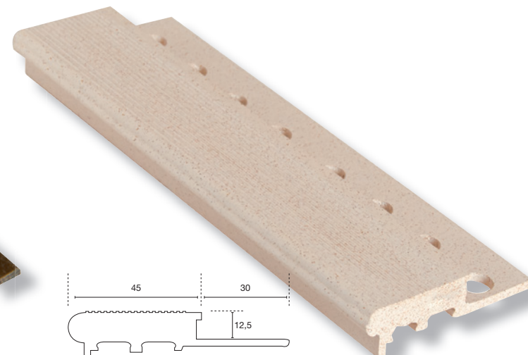
PELDAÑO RÚSTICO 12,5x45 MM. RUSTIC STEP-TREAD 12,5x45 MM.
