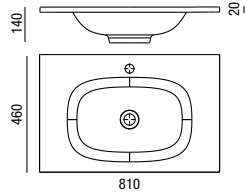
Lavatório BARI 810 x 20 x 460 mm
