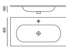
Lavatório NAPOLI 1010 x 20 x 455 mm
