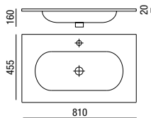
Lavatório NAPOLI 810 x 20 x 455 mm
