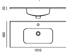
Lavatório MONZA 1010 x 20 x 460 mm
