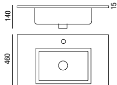
Lavatório SQUARE 810 x 15 x 460 mm
