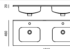
Lavatório MONZA doble 1210 x 20 x 460 mm
