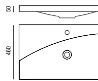
Lavatório AMALFI 1010 x 50 x 460 mm
