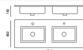
Lavatório SQUARE doble 1210 x 15 x 460 mm
