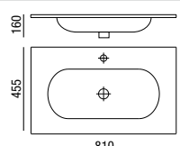
Lavatório NAPOLI 810 x 20 x 455 mm
