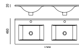
Lavatório IBERIA doble 1205 x 20 x 460 mm
