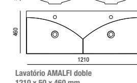
Lavatório AMALFI doble 1210 x 50 x 460 mm
