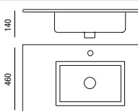
Lavatório SQUARE 1010 x 15 x 460 mm
