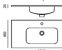
Lavatório MONZA 1010 x 20 x 460 mm
