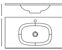
Lavatório BARI 1010 x 20 x 460 mm
