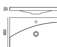
Lavatório AMALFI 810 x 50 x 460 mm
