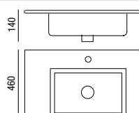
Lavatório SQUARE 810 x 15 x 460 mm
