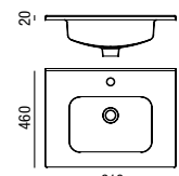
Lavatório MONZA 610 x 20 x 460 mm
