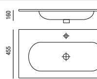
Lavatório NAPOLI 1010 x 20 x 455 mm
