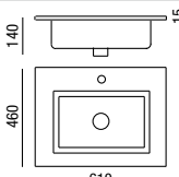
Lavatório SQUARE 610 x 15 x 460 mm
