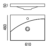
Lavatório AMALFI 610 x 50 x 460 mm
