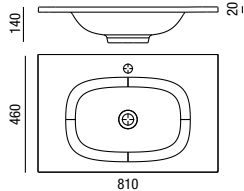
Lavabo BARI 810 x 20 x 460 mm
