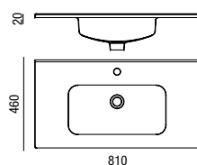
Lavabo MONZA 810 x 20 x 460 mm
