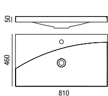
Lavabo AMALFI 810 x 20 x 460 mm
