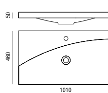
Lavabo AMALFI 1010 x 20 x 460 mm
