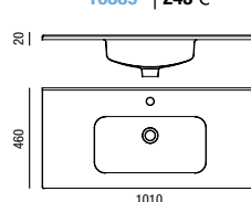
Lavabo MONZA 1010 x 20 x 460 mm
