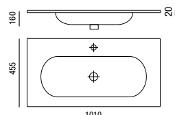
Lavabo NAPOLI 1010 x 20 x 455 mm
