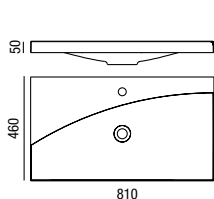
Lavabo AMALFI 810 x 50 x 460 mm
