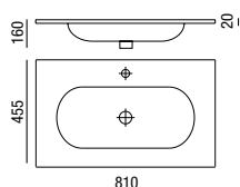
Lavabo NAPOLI 810 x 20 x 455 mm
