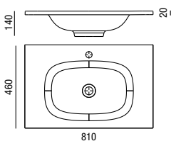
Lavabo BARI 810 x 20 x 460 mm
