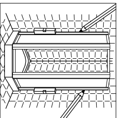
3. Úprava celku na sprchové vaničce. Srovnejte podle vodováhy dveře a boční stěny. Pokud není sprchová vanička dokonale vodorovná, vyprodíže celou sprchu, aby se tato závada odstranila. Vyznačte sponou vyrovnávací profilu obou bočních stěn.
