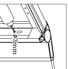
9. Vyměňte v podlahovém otvoru díru o Ø 3 mm a zasroubujte kryt dveří a bočních stěn pomocí šroubu 3,5 x 5,5 mm.
