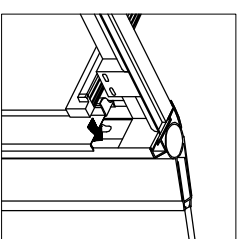
11. Srovnejte všechny prvky, proveďte jejich náležitý chod a utáhněte definitivně všechny šrouby.
