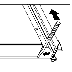
7. Vyměňte profil krytu rámu pomocí plochého šroubováku.
