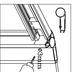
12. Ve vzdálenosti asi 100 mm od horního a dolního kraje vyměňte otvor o Ø 3 mm do spojovacího profilu a krytu boční stěny. Zajištěte celou pomocí šroubu 3,5 x 9,5 mm.
