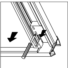
1. Odsřobuje držák otočného čepu a vyměje dveře z krytu.
