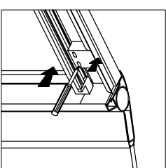
10. Opět namontujte prvek nebo prvky dveří do rámu a upevněte držák čepu.
