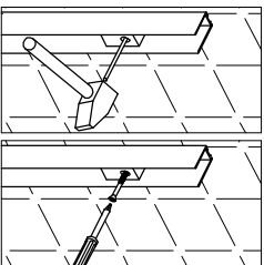
4. Vyměňte vyrovnávací profil z bočních stěn s tím, že se částičně uvoří boční šrouby. Srovnejte jejich polohu podle značek, a vyznačte si polohu pro otvory k vyvrtání.
