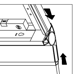
8. Sešroubujte rám a boční stěny a srovnejte je s krajem sprchové vaničky.
