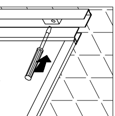
6. Upevněte vyrovnávací profil pomocí šroubů Ø 4,2 x 60 mm. Ujistěte, že boční stěny do vyrovnávacího profilu.
