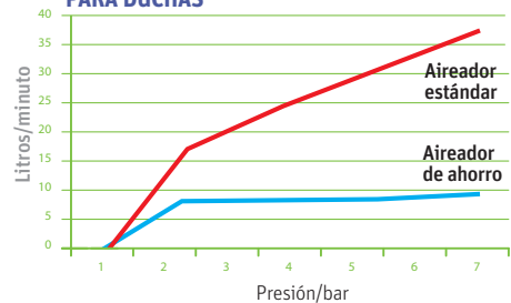
GRÁFICA COMPARATIVA DE CAUDALES PARA DUCHAS
