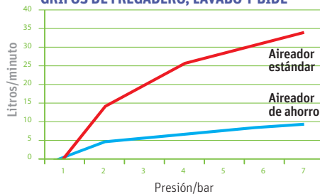
GRÁFICA COMPARATIVA DE CAUDALES PARA GRIFOS DE FREGADERO, LAVABO Y BIDÉ
