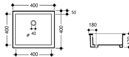
Lavabo Quadratta / Quadratta Washbasin
