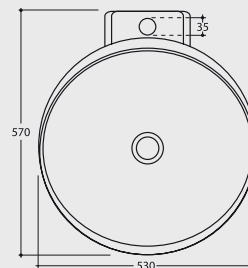
MELAORZ57LT Lavabo porcelana "ORIZZONTE-57" latino bianco-nero ORIZZONTE-57 ceramic washbasin
