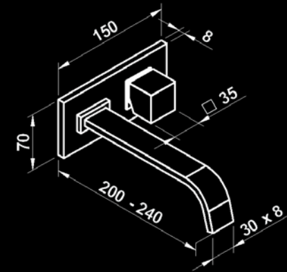
ref. SI46265 Batería Lavabo Pared DREAM Cromo
