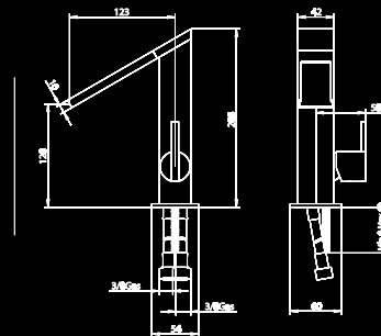
BA78032-00 DIVE BAJO Contiene desagüe clicker con tapón cuadrado
