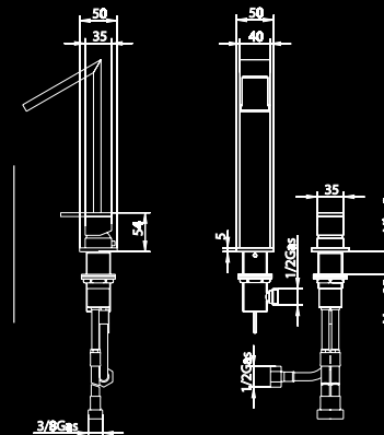
BA78032-00 DIVE ALTO Contiene desagüe clicker con tapón cuadrado + Prolongador ref. BA91954
