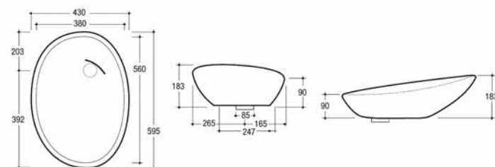
Lavabo mod. BIKO
