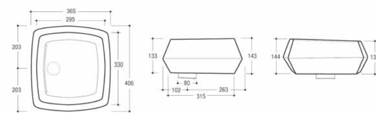
Lavabo mod. HASANA
