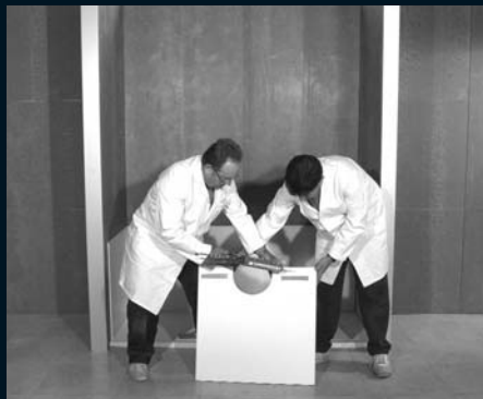
16. siliconamos panel corto de grifería y aplicamos adhesivo a dos caras
