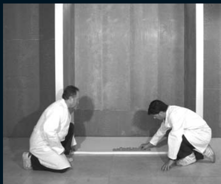
8. nivelamos el plato
