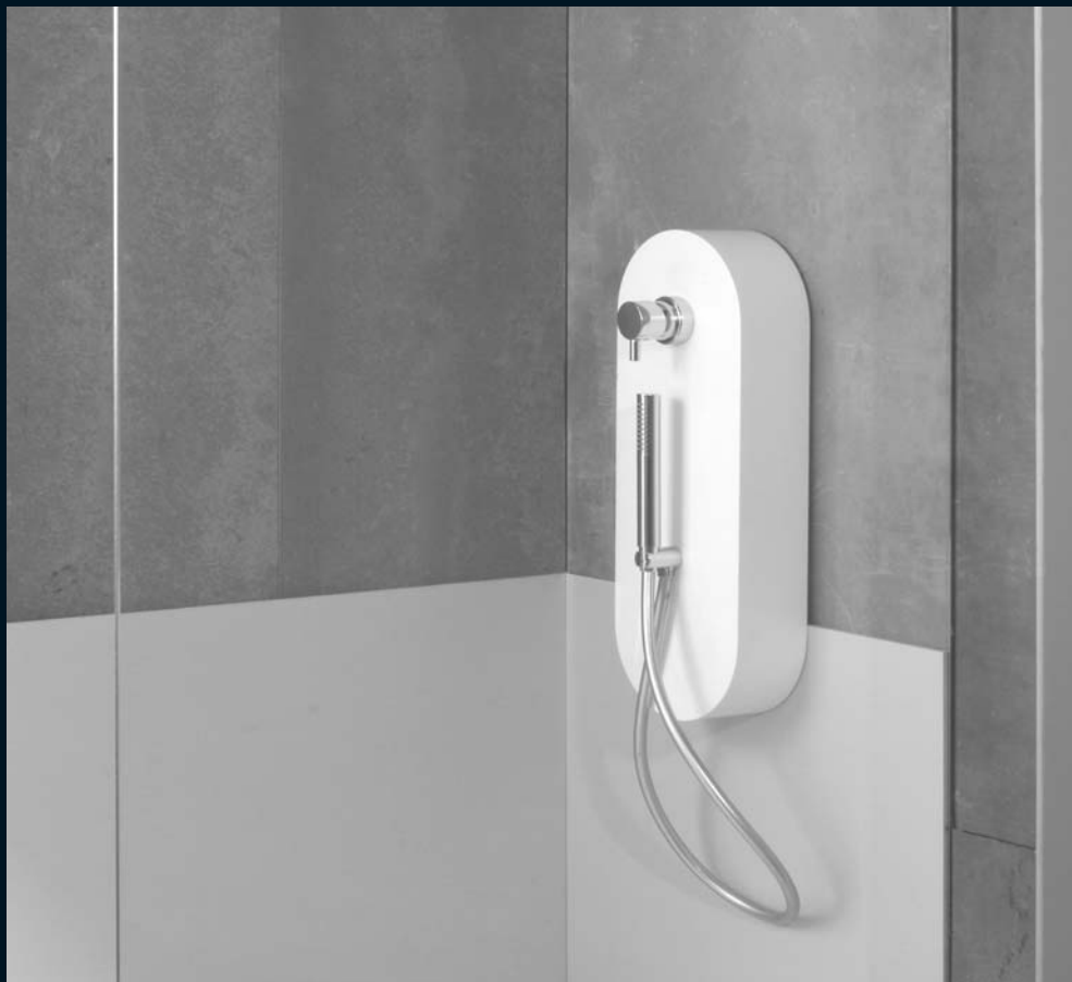
h-1 detalle panel porcelánico de 3mm beige (opción 30 colores) con caja de grifería
