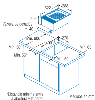
Modelo: 3EB-6030 L
