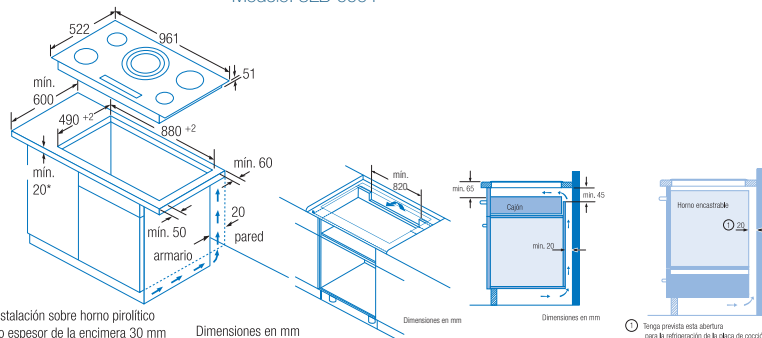
Modelo: 3EB-990 F
