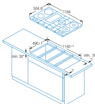
Medidas para unión de cuatro placas
