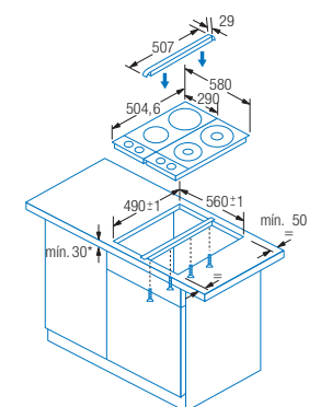
Medidas para unión de dos placas
