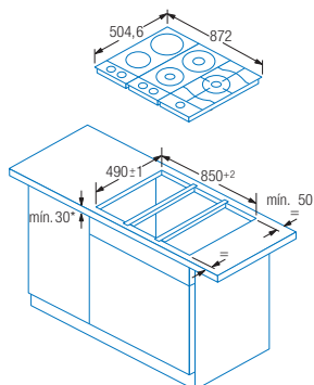
Medidas para unión de tres placas
