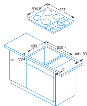
Medidas para unión de una placa de 60 cm y una placa modular.
