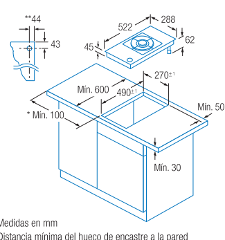
Modelos: 3EB-2030 LB y 3EB-1030 LB
