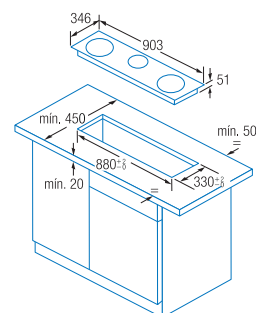
Modelo: 3EB-928 L
