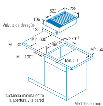
Modelo: 3EB-4030 L
