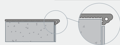
CARTABÓN FIORENTINO 33 x 33 x 3 cm
